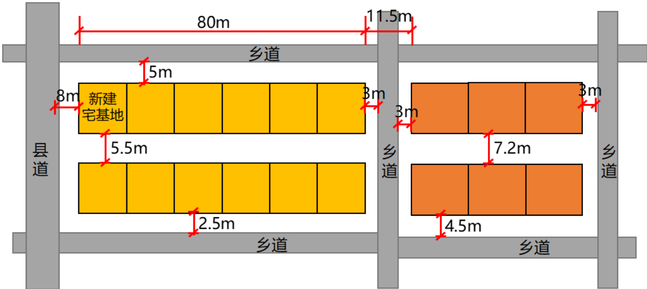
集中连片式村民建房建设管控指引图
