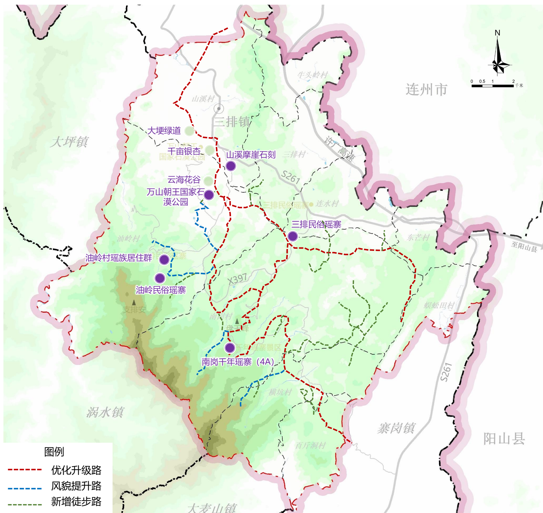
三排镇交通体系规划图
