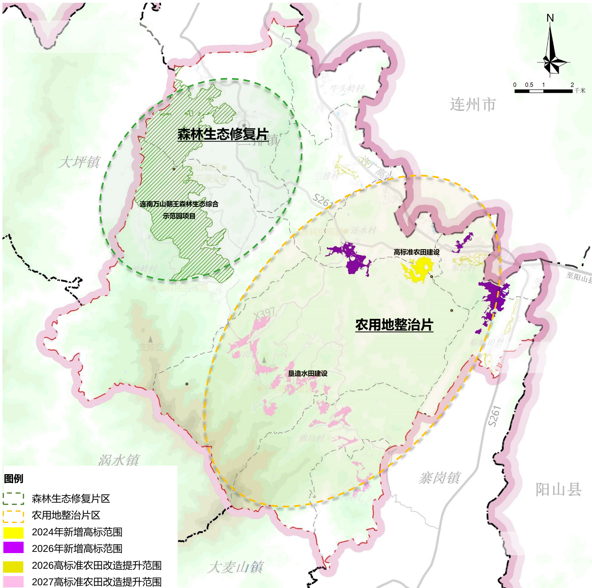
三排镇农用地整理规划布局图
