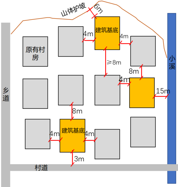
插花式村民建房建设管控指引图
