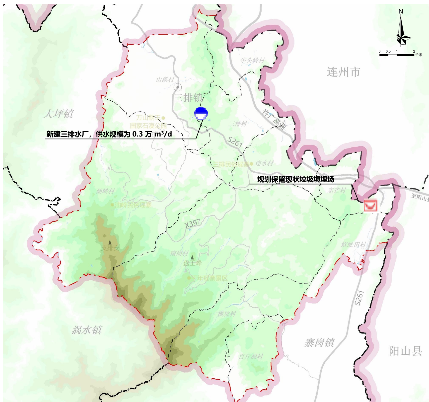
三排镇重大市政基础设施布局图
