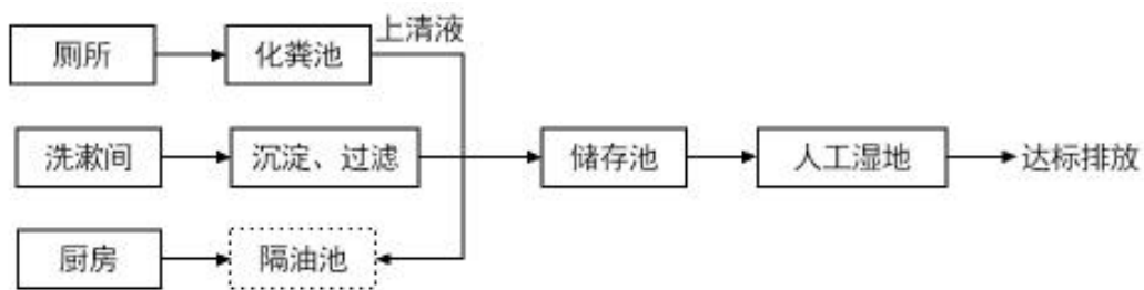
图 4-4 三格化粪池/沼气池-人工湿地/生态塘工艺流程图
