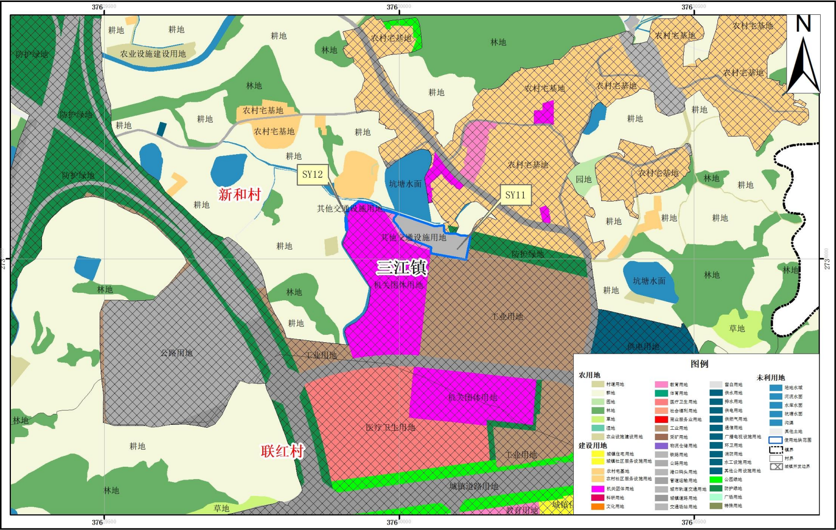
清远市连南瑶族自治县三江镇使用后地块土地使用规划局部图（SY11-12）
